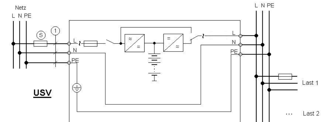
Abb. 4: Anschluss der USV
