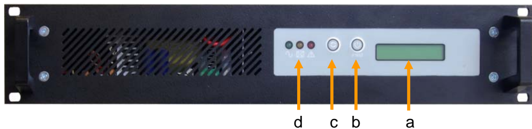
Abb. 2: Frontansicht MD 700/1000/1500 RM
