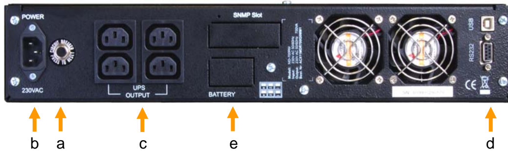
Abb. 3: Rückwand-Ansicht MD 700/1000/1500 RM
