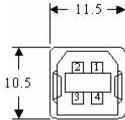
Abb. 12: Pinbelegungen der USE Karte
