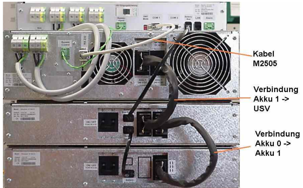
Abb. 18: Verbindung von USV, der Akku- bank und des Bypassschalters (optional).
