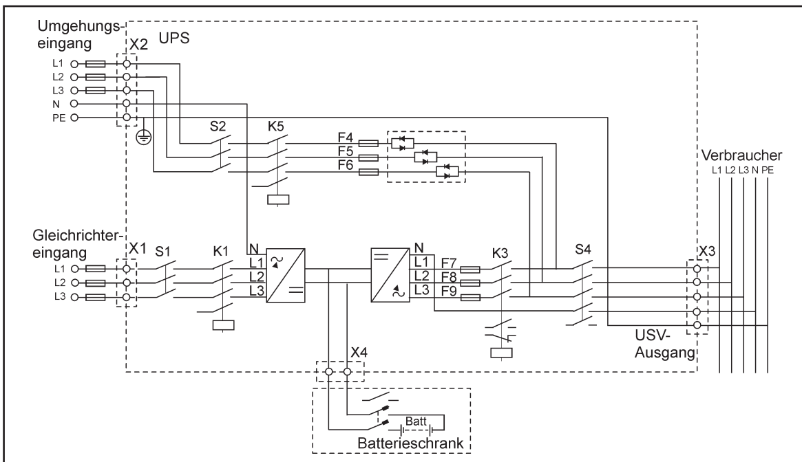
Abb. 6 USV-Anlage 100 – 160 kVA im Fünfleiternetz
