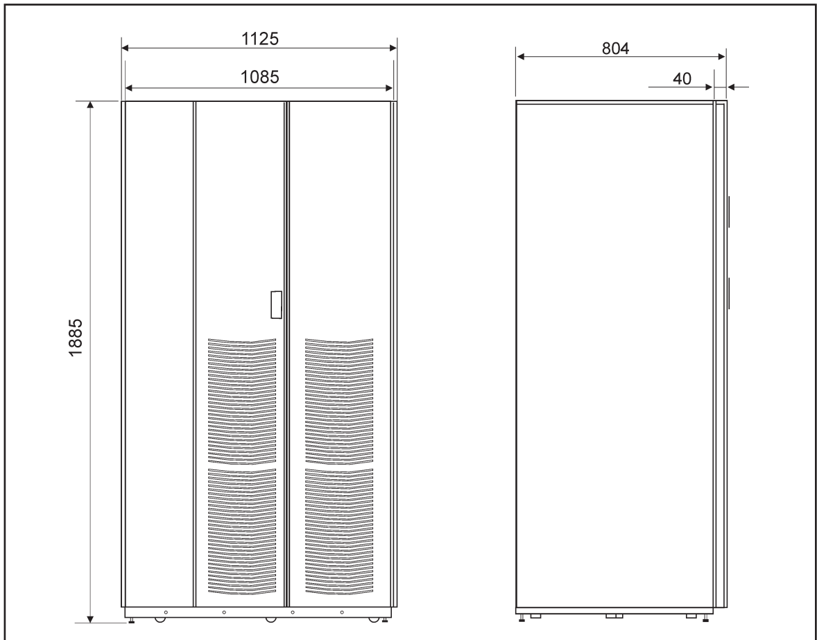
Abb. 43 Abmessungen - Batterieschrank
