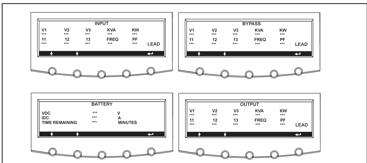
Abb. 25 Anzeigefenster für Eingangs-, Umgehungs-, Batterie- und Ausgangsdaten
