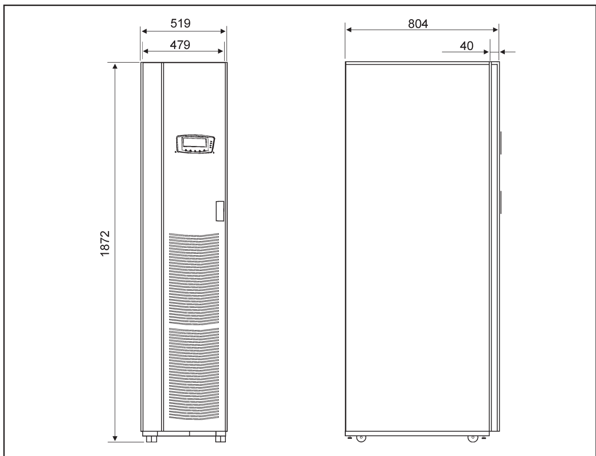
Abb. 39 Abmessungen – USV-Schrank (40-80 kVA)
