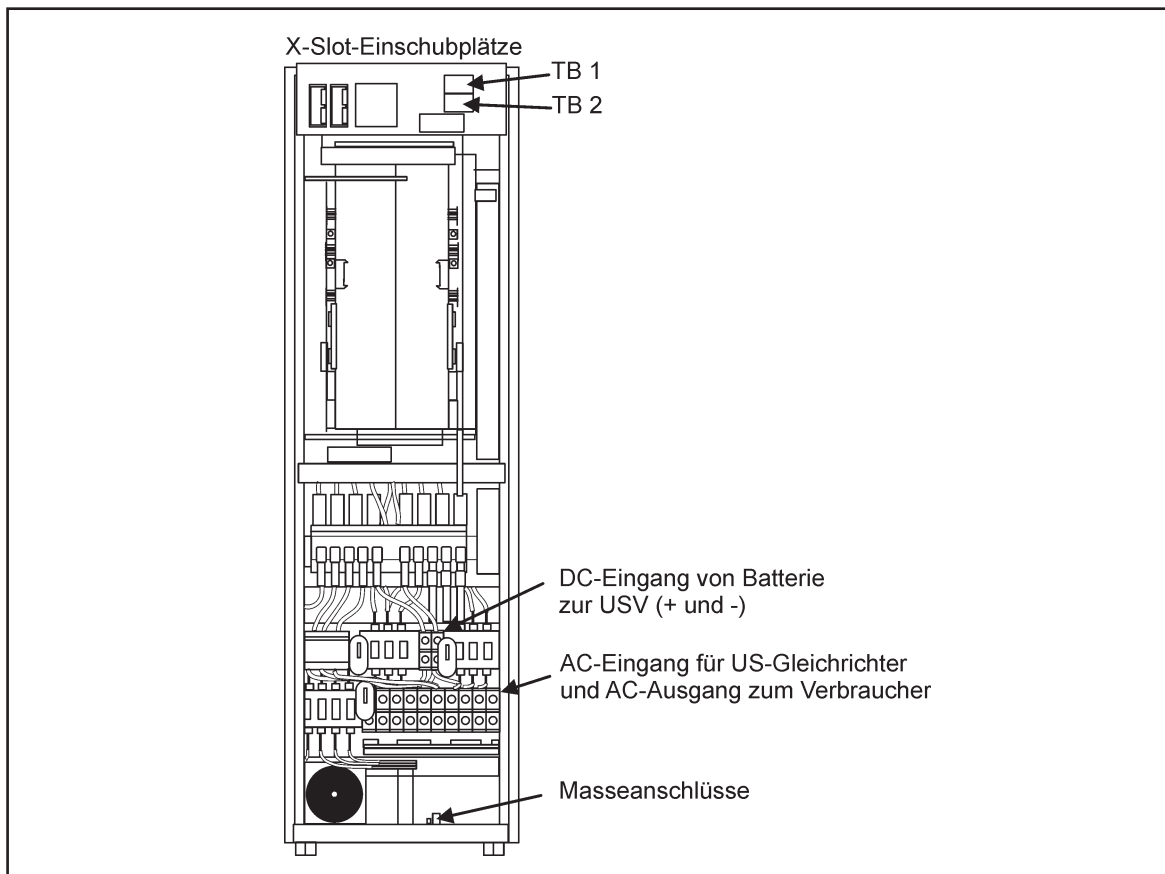
Abb. 4 Versorgungs- und Signalanschlüsse an der USV-Einheit
