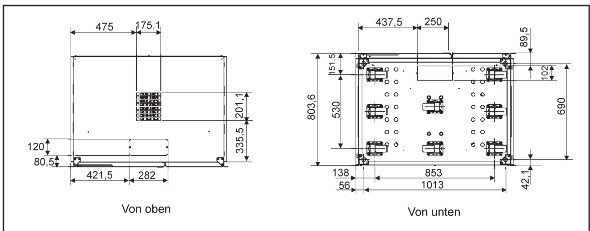
Abb. 44 Batterieschrank – Abmessungen oben und unten
