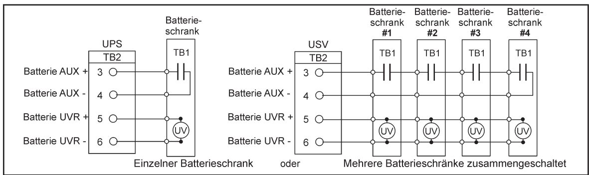
Abb. 13 AUX- und UVR-Verdrahtung der Batterie
