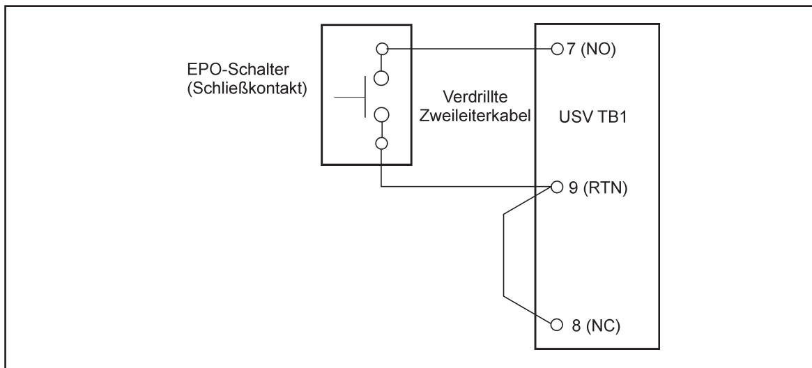
Abb. 21 Anschlussplan für Fernabschaltung
