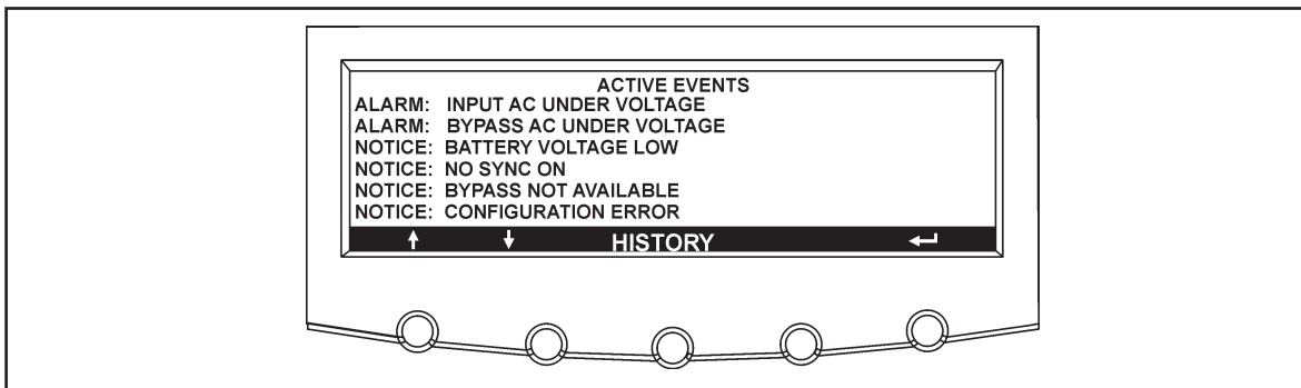
Abb. 24 Keine Synchronisation. Umgehung nicht verfügbar.
