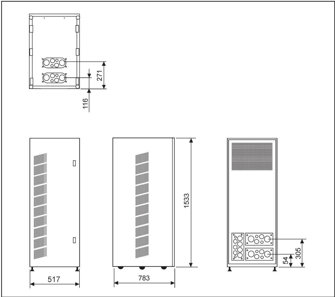
Abb. 45 HotSync-Parallelschaltsschrank (SPM9390-80kVA-4UPS) – Abmessungen )
