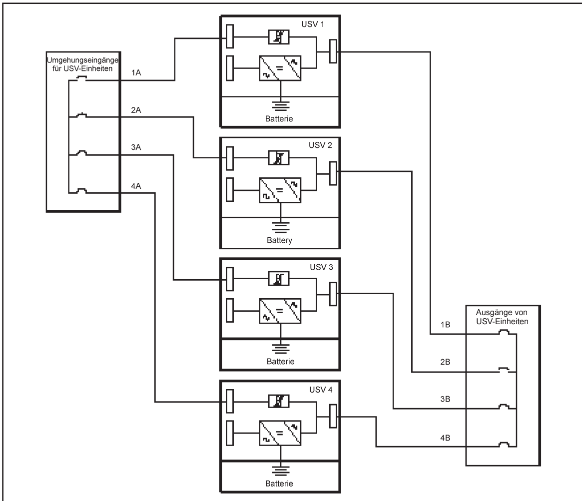
Abb. 34 Schaltplan für Verkabelung mehrerer USV-Einheiten und relative Kabellängen
