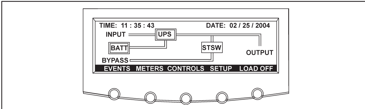
Abb. 30 Grafisches Fenster und Hauptmenü
