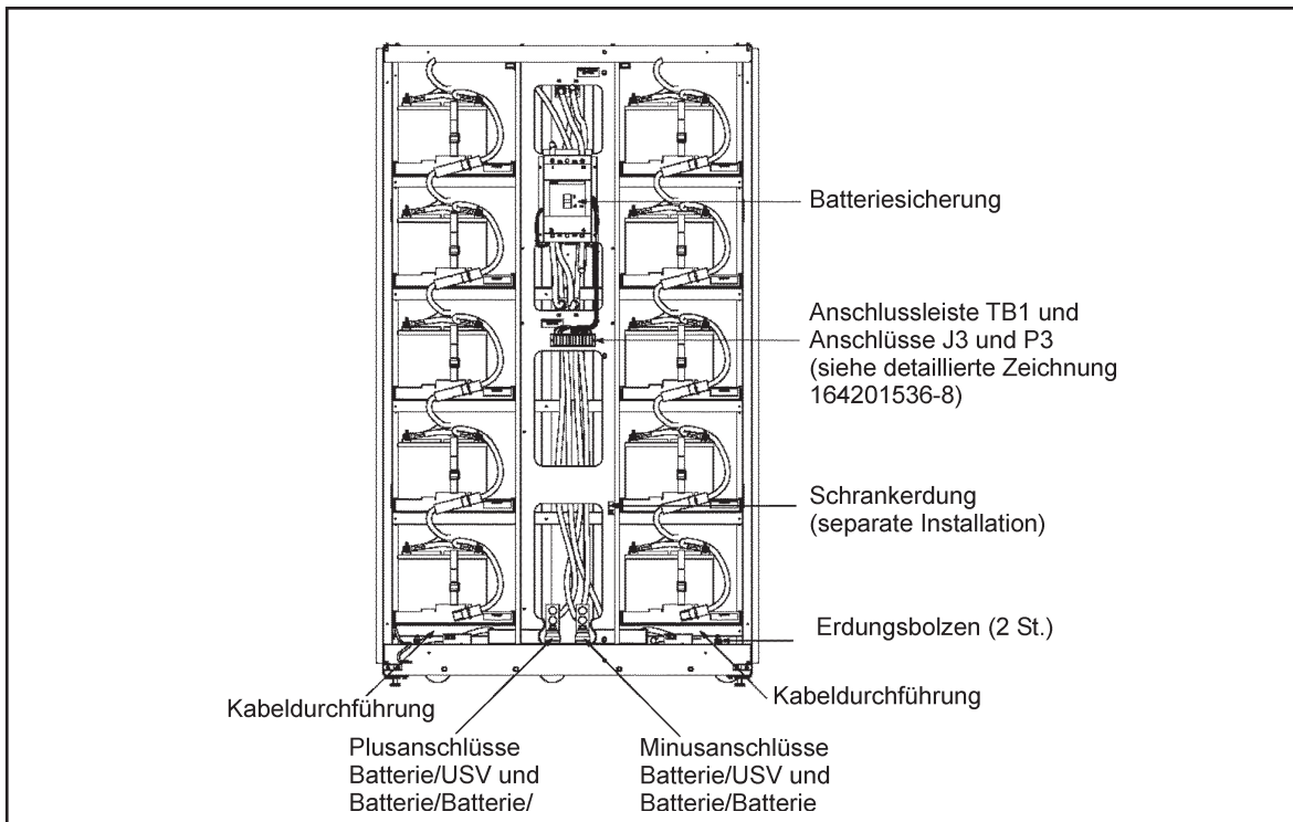
Abb. 8 Batterieschrank mit offener Türe – die Anschlüsse sind zu sehen
