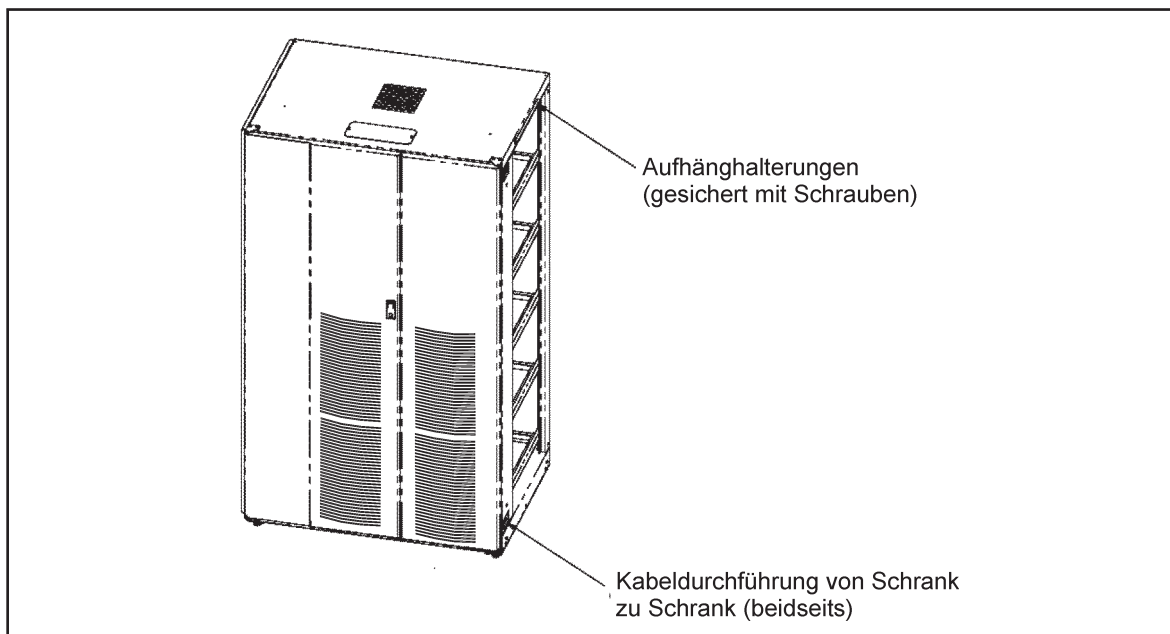
Abb. 11 Aufhängehalterungen am Batterieschrank
