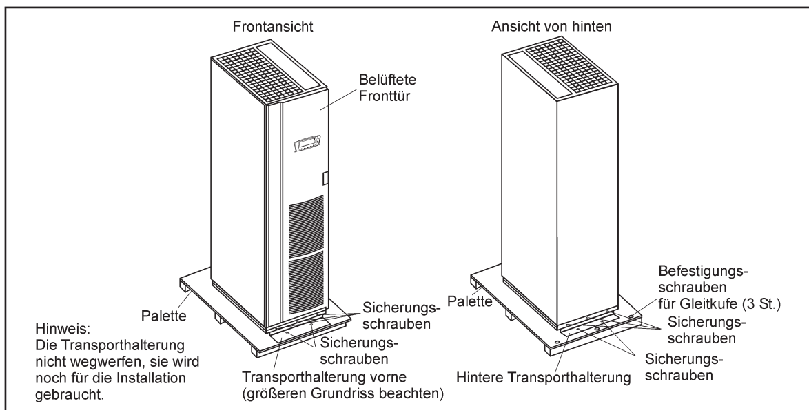
Abb. 3 Entfernen der Sicherungsschrauben und Transporthalterungen
