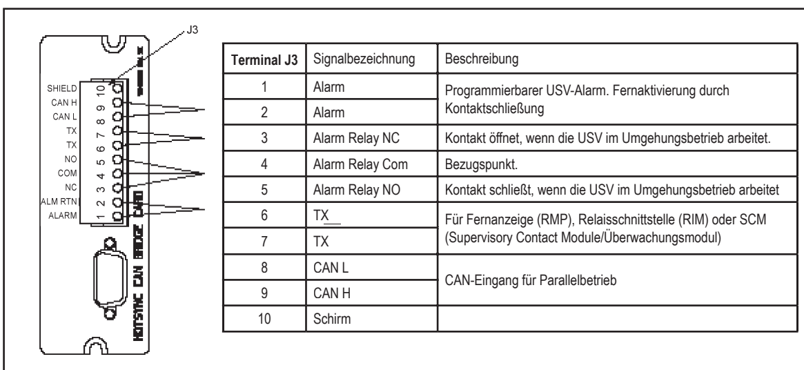
Abb. 35 CAN-Bus-Karte mit Anschlüssen
