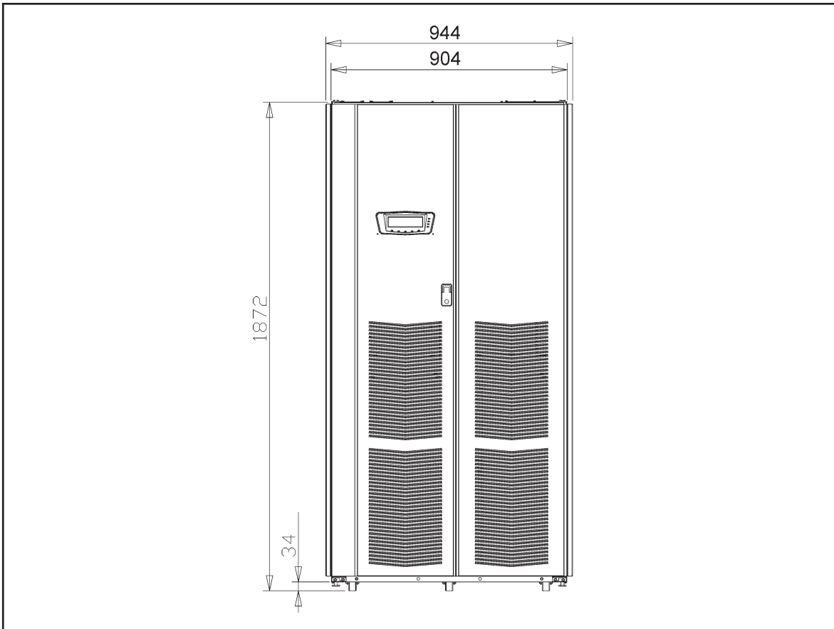
Abb. 41 Abmessungen – USV-Schrank (100-160 kVA)
