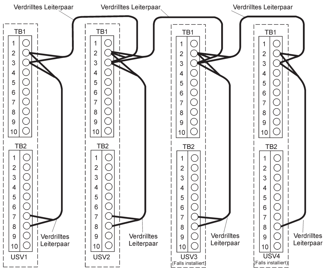
Abb. 38 Signalverkabelung für die Umgehung, HotSync-Systeme
