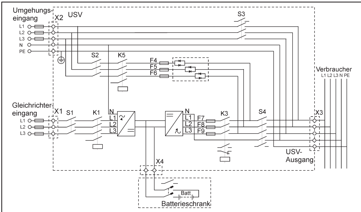
Abb. 5 USV-Anlage 40 – 80 kVA im Fünfleiternetz
