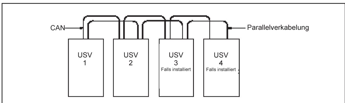
Abb. 37 Parallele Signalverkabelung des HotSync-Systems
