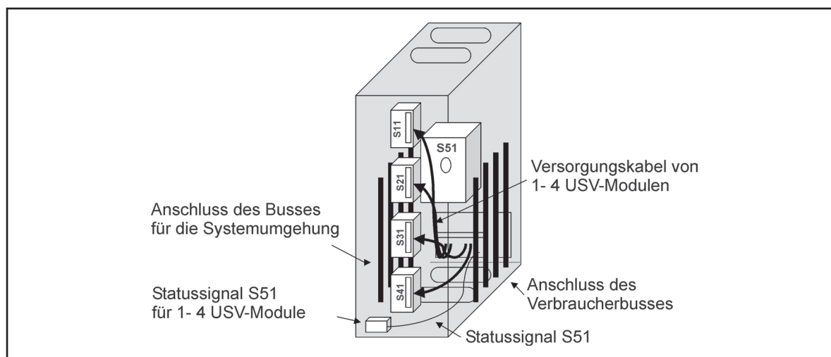
Abb. 32 Kabelverlegung für SPM9390-80kVA-4UPS
