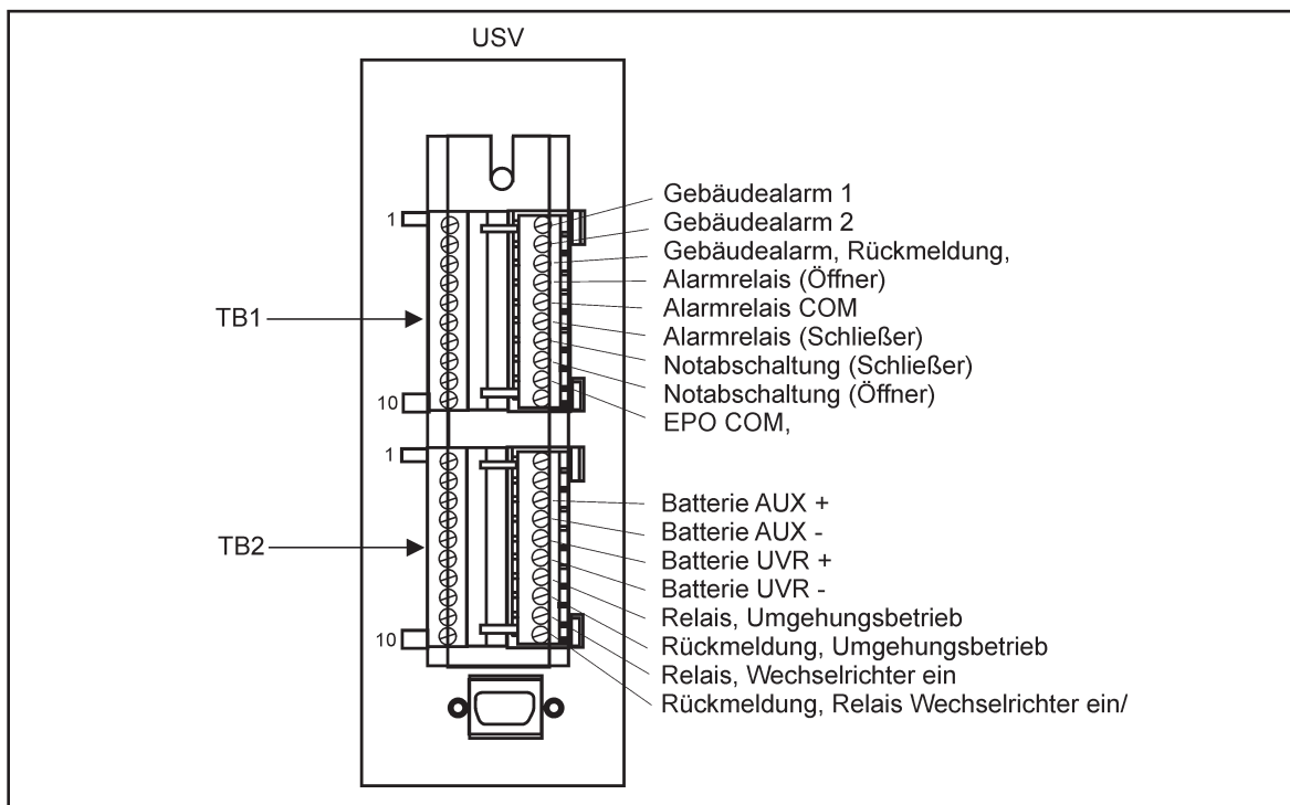
Abb. 19 Eingänge und Ausgänge
