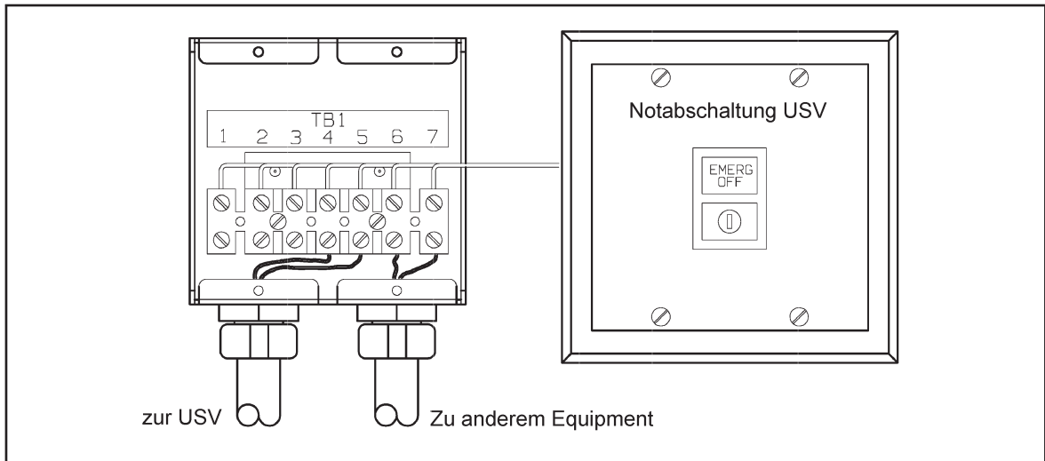
Abb. 20 Beispiel für die Einrichtung einer Notabschaltung (EPO)
