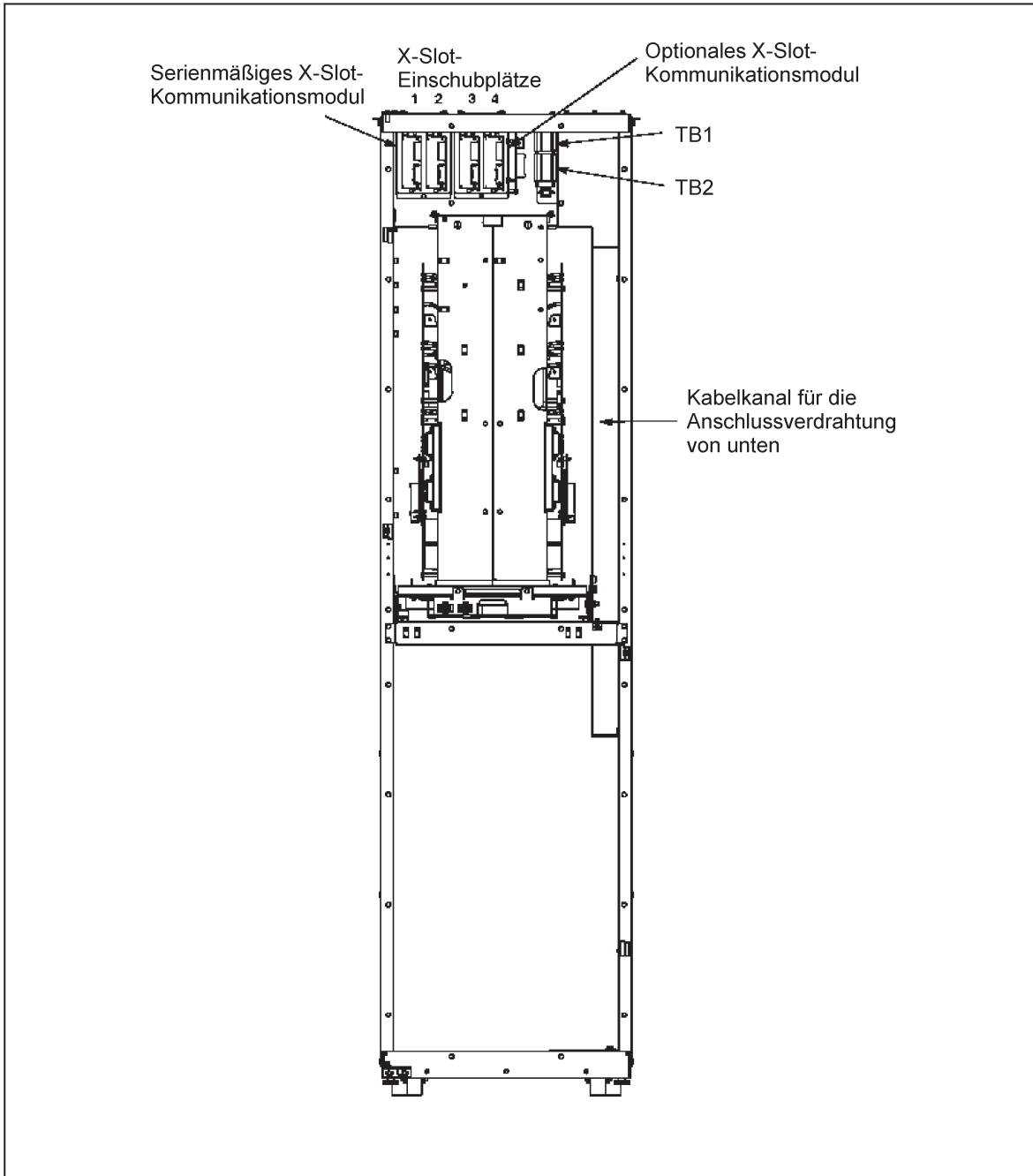
Abb. 17 Kommunikationsschnittstelle
