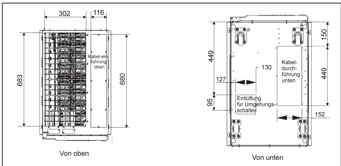
Abb. 40 USV-Schrank – von oben und unten (40-80 kVA)
