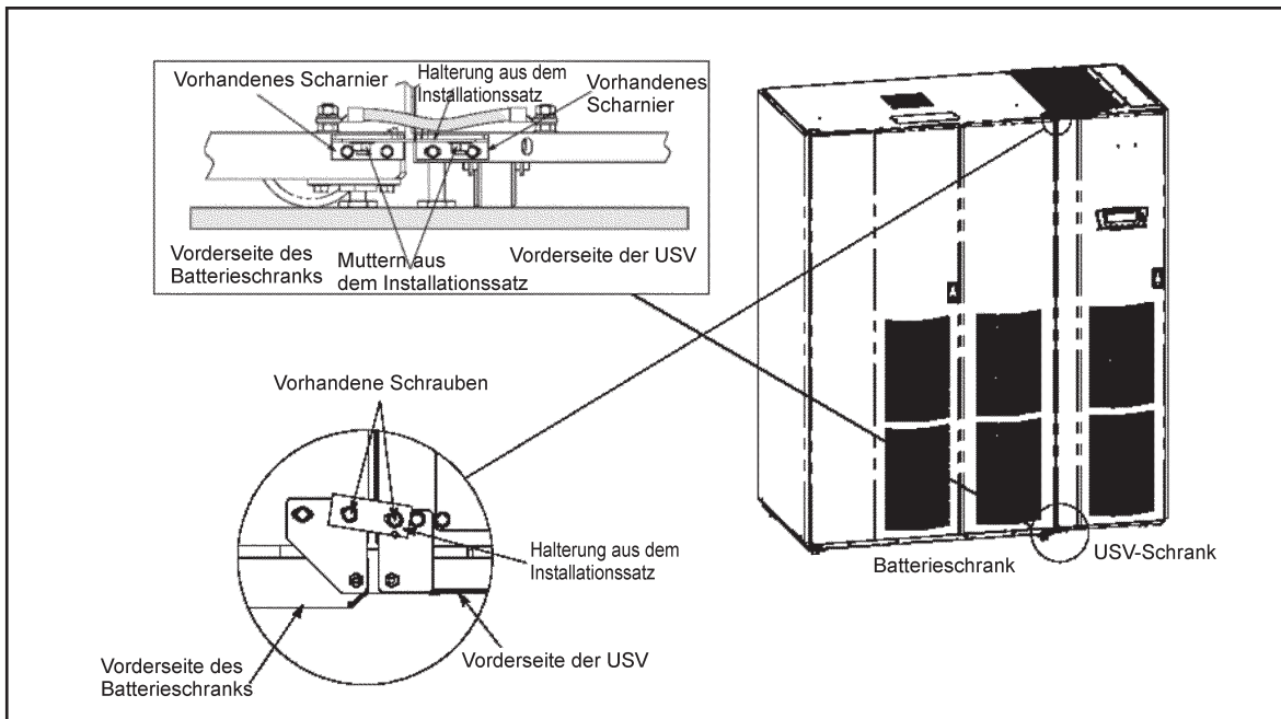
Abb. 10 Befestigung des Batterieschranks an der USV-Einheit
