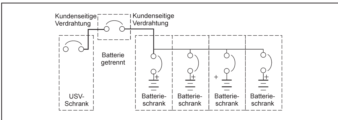
Abb. 16 Separat von der USV aufgestellte Batterieschränke
