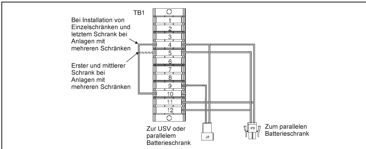
Abb. 14 TB1-Verbindung
