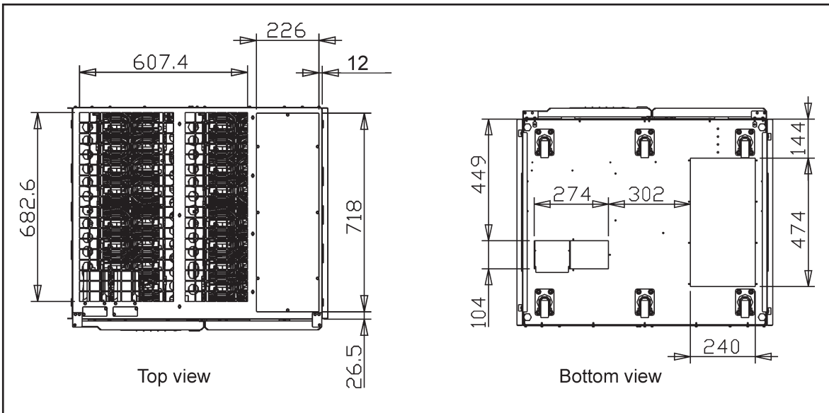
Abb. 42 USV-Schrank – von oben und unten (100-160 kVA)
