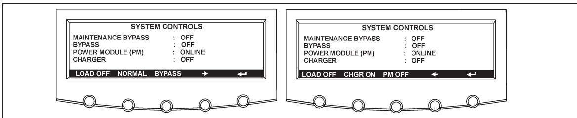
Abb. 26 Fenster 1 und 2 für die Systemsteuerung
