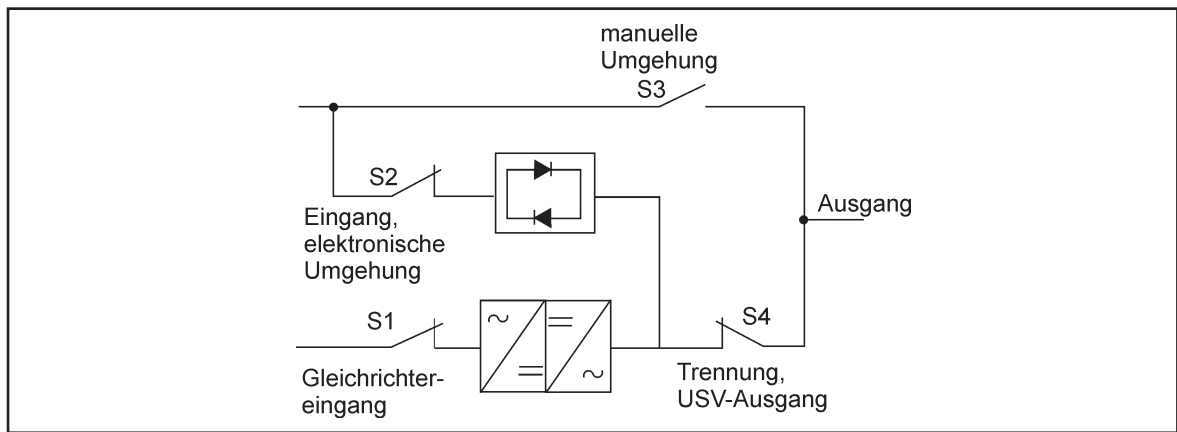
Abb. 31 Normale Stellung der vier MBS-Schalter
