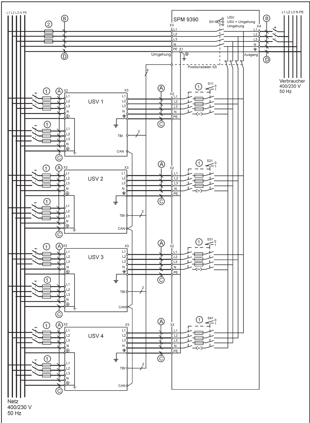
Abb. 33 Anschlussplan für HotSync-Parallelsystem mit vier USV-Modulen und Parallelschalt-schrank
