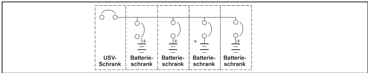
Abb. 12 Elektrische Verbindung des Batterieschranks – allgemein
