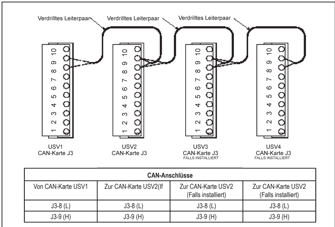
Abb. 36 CAN-Verkabelung für Parallelsystem
