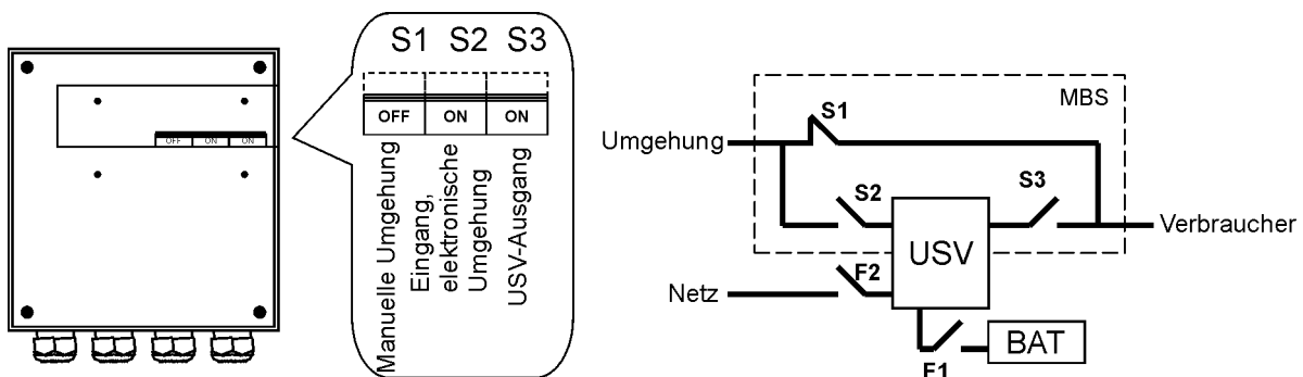
Abb. 36. Servicestellung der drei MBS-Schalter (Verbraucher wird über Umgehung versorgt)
