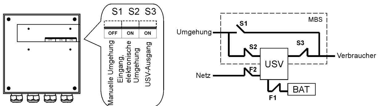
Abb. 35. Normale Stellung der drei MBS-Schalter (im USV-Betrieb)
