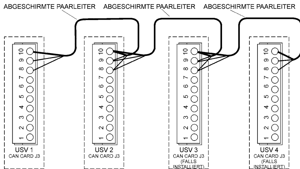
VERDRAHTUNG DER CAN-KARTEN IN PARALLELSYSTEMEN
