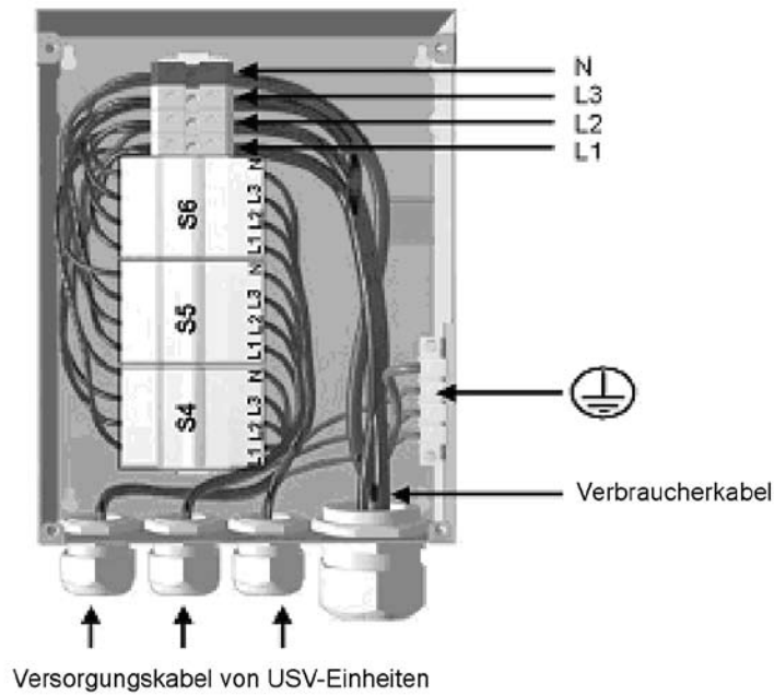
Abb. 39. Kabelführung im Systemparallelmodul
