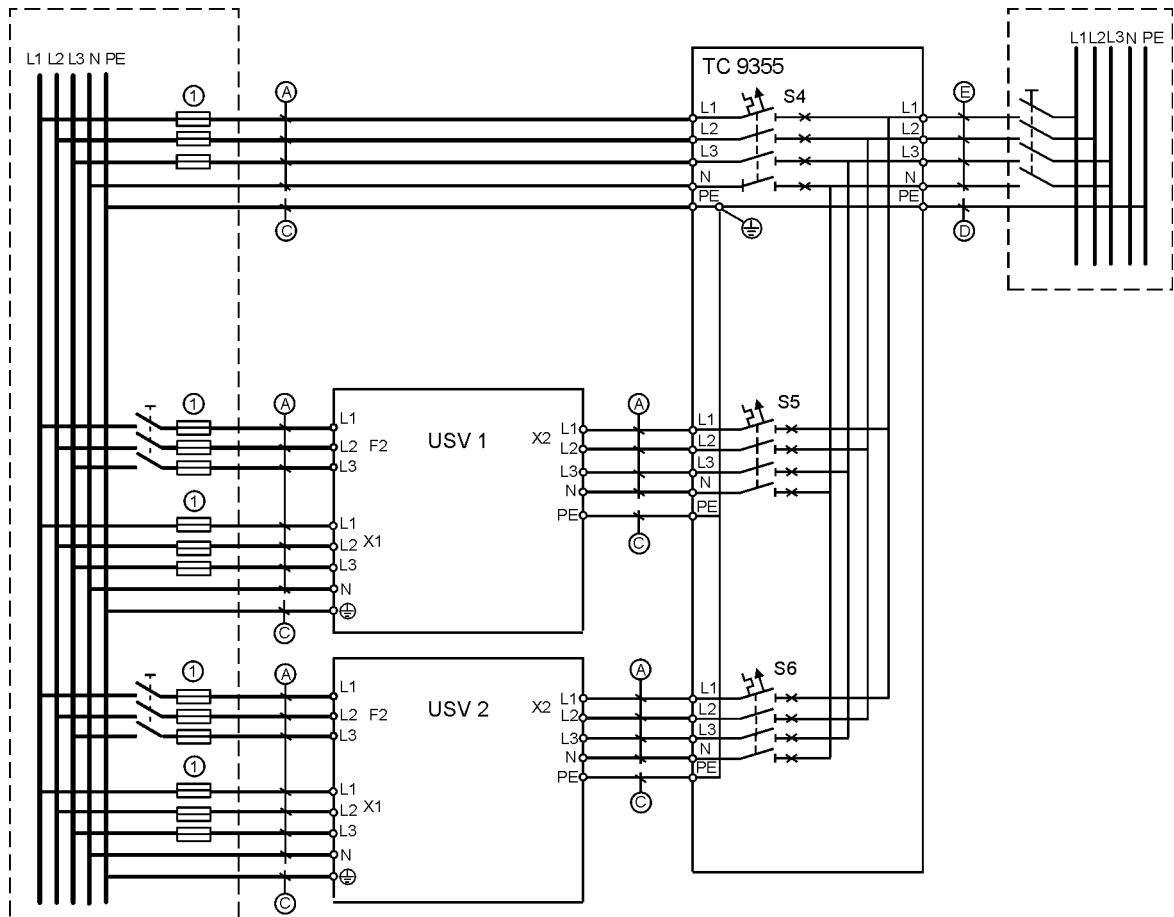
Abb. 41. Systemparallelmodul – Schaltplan für 2 USV-Einheiten und Umgehung
