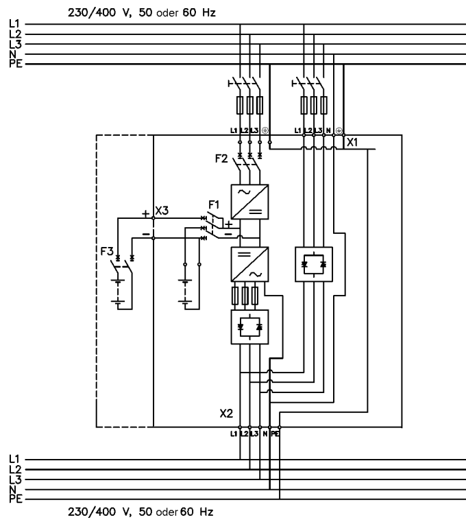
Abb. 16. Schaltplan für USV N-Modell
