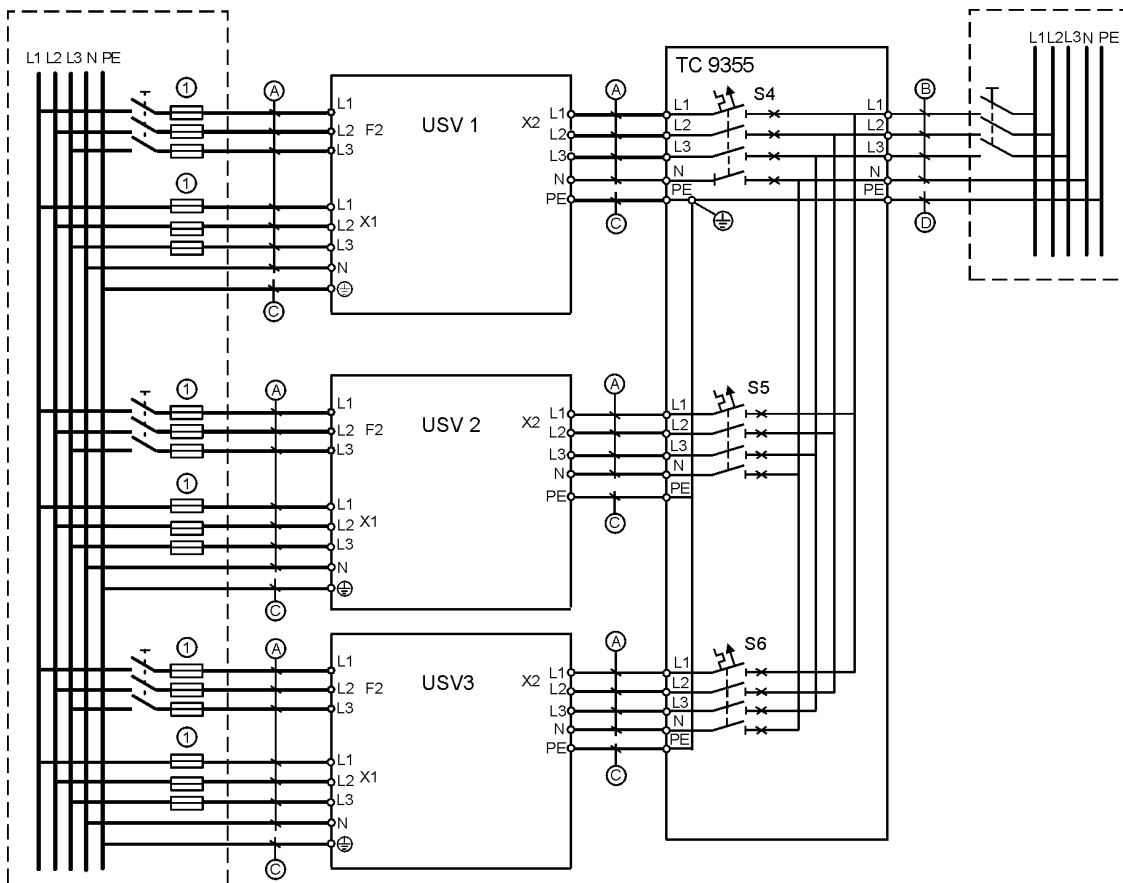
Abb. 39. Kabelführung im Systemparallelmodul
