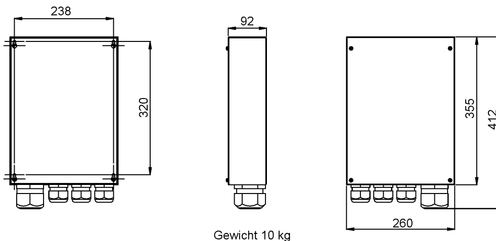
Abb. 38. Abmessungen des Systemparallelmoduls
