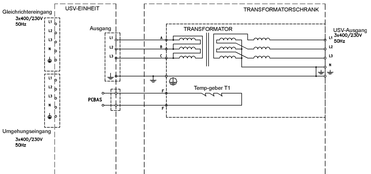
Abb 10. Optionaler Trenntransformator – werkseitig eingebaut oder separat zum Nachrüsten
