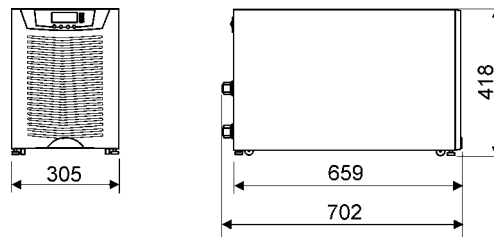
Abb. 47. USV-Modelle ohne Batterieschränke
