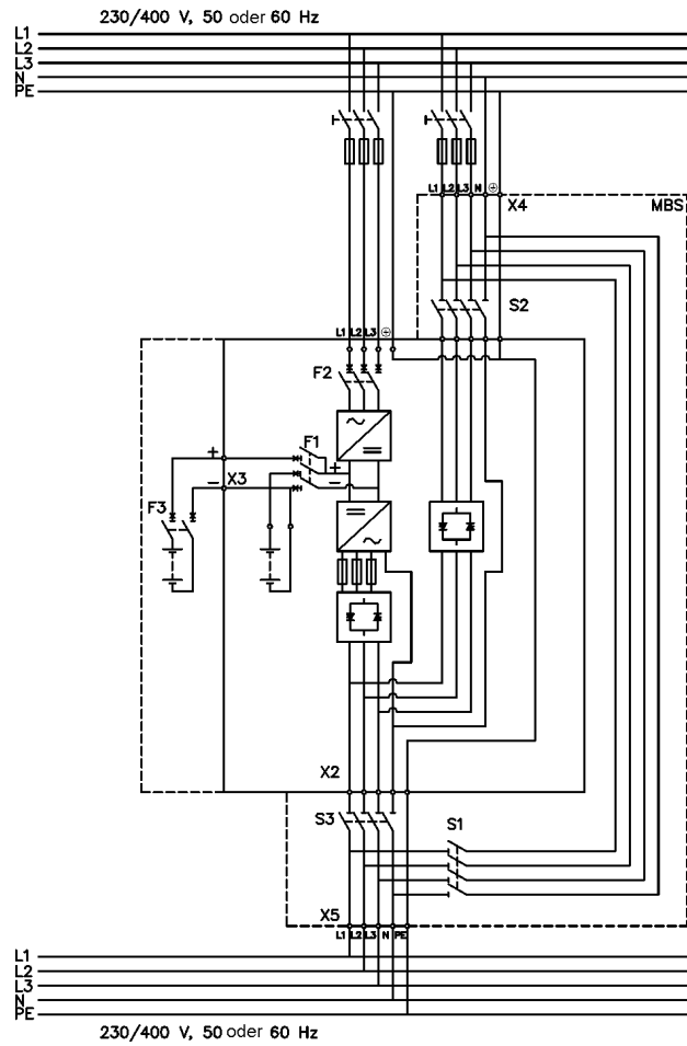
Abb. 15. Schaltplan für USV N-Modell mit eingebautem MBS
