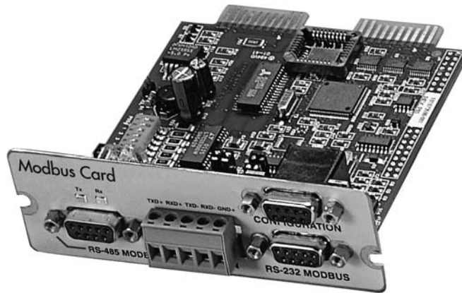
Abb. 27. Modbus/Jbus-Modul
