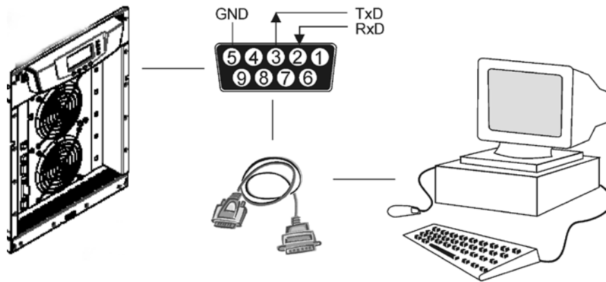
Abb. 21. Schnittstellenbelegung
