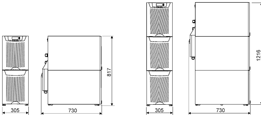
Abb. 49. USV-Modelle mit Batterieschränken und installiertem MBS
