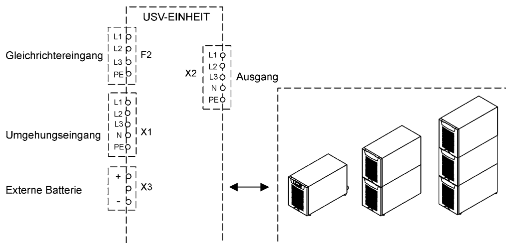
Abb. 13. Versorgungsanschlüsse an USV-Einheiten
