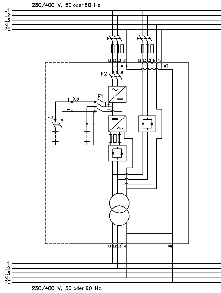
Abb. 17. Schaltplan für USV NT-Modell
