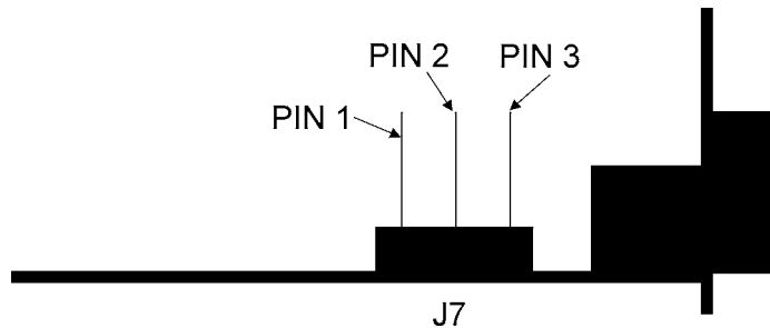
Abb. 46 Brücke J7 an der CAN-Karte – Kein Abschlusswiderstand: Stift 2 – 3 überbrückt. Mit Abschlusswiderstand: Stift 1 – 2 überbrückt.
