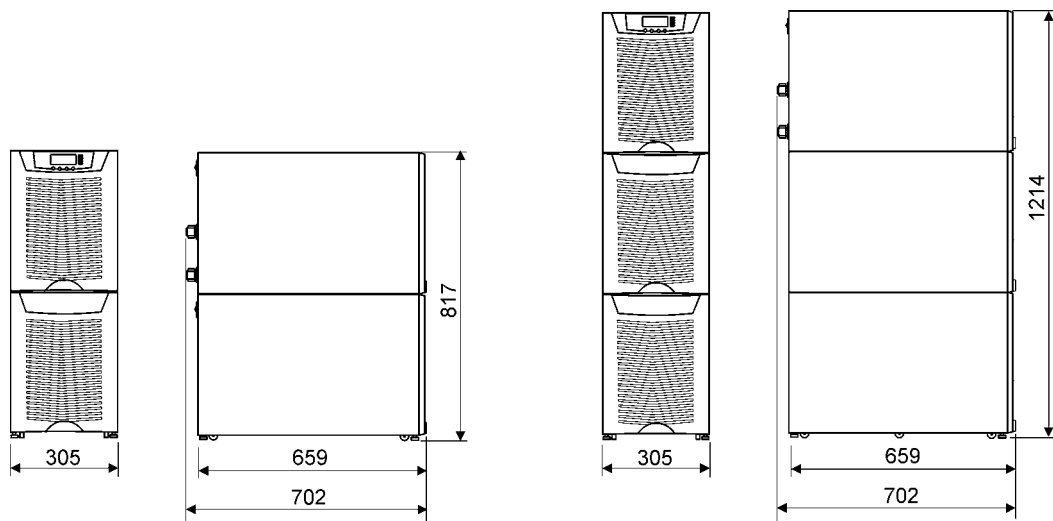
Abb. 48. USV-Modelle mit Batterieschränken
