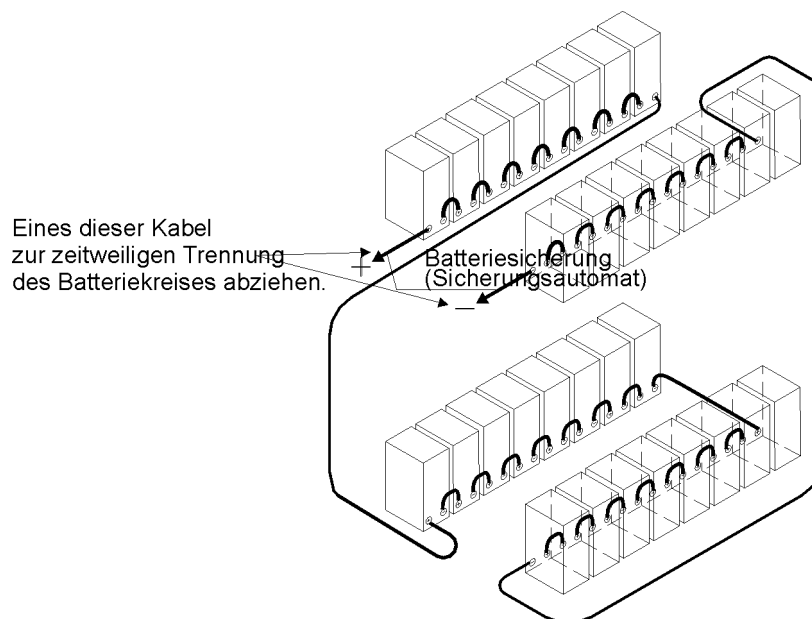
Abb. 19. Sicherheitshalber das Plus- oder Minuskabel des Batteriekreises trennen, bevor USV und externer Batterieschrank verbunden werden
