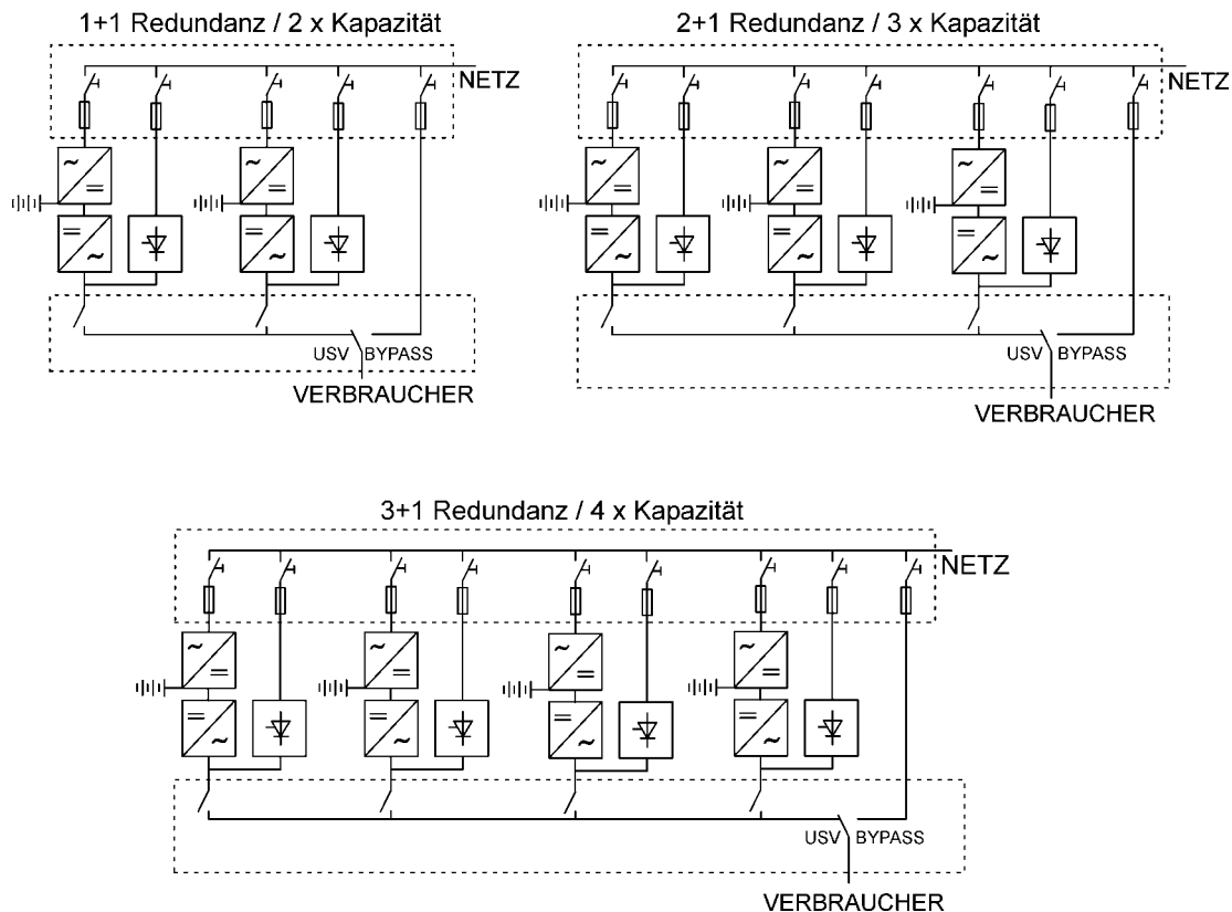
Abb. 37 Parallelkonfigurationen mit USV-Modulen
