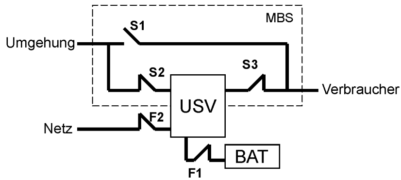
Abb. 34. Normale Stellung der drei MBS-Schalter
