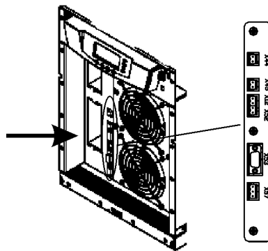
Abb. 20. Anschlüsse für Kommunikationskabel: Signaleingänge (X44 & X45); Notabschaltung (EPO, NC (X12) & NO (X52)); RS-232 (X53); Relaisausgang (X57)
