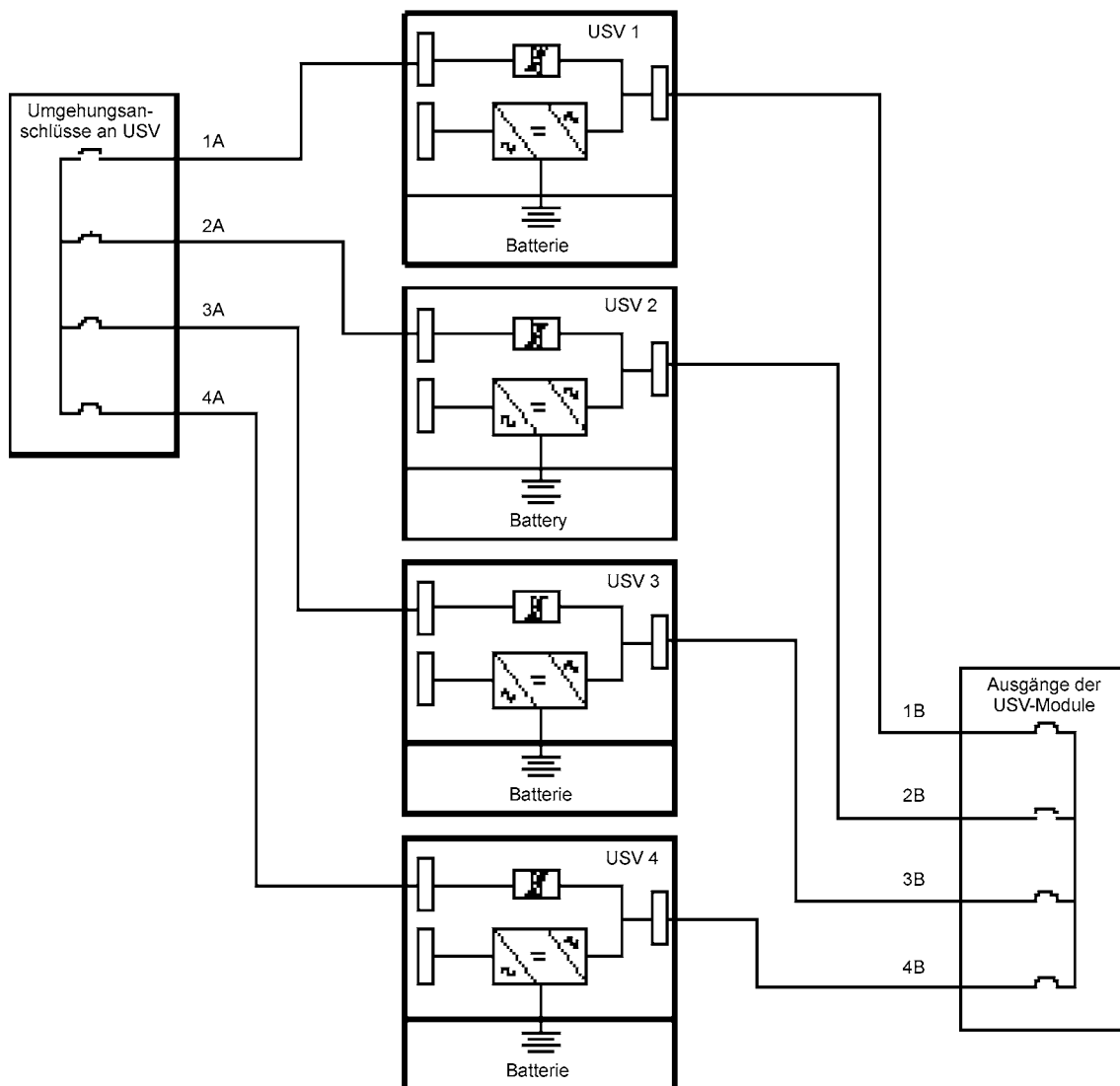
Abb. 43 Anschlussplan für Umgehung sowie Kabelführung
