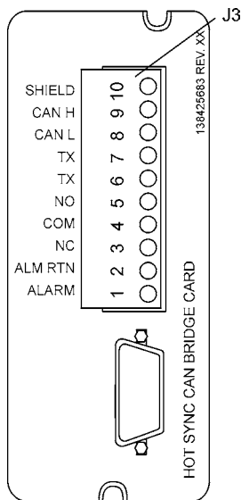
Abb. 44 HotSync X-Slot-Adapter und Anschlussleiste
