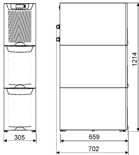
Abb. 51. USV-Modell mit Batterieschrank (Mitte) und Transformator (unten)
