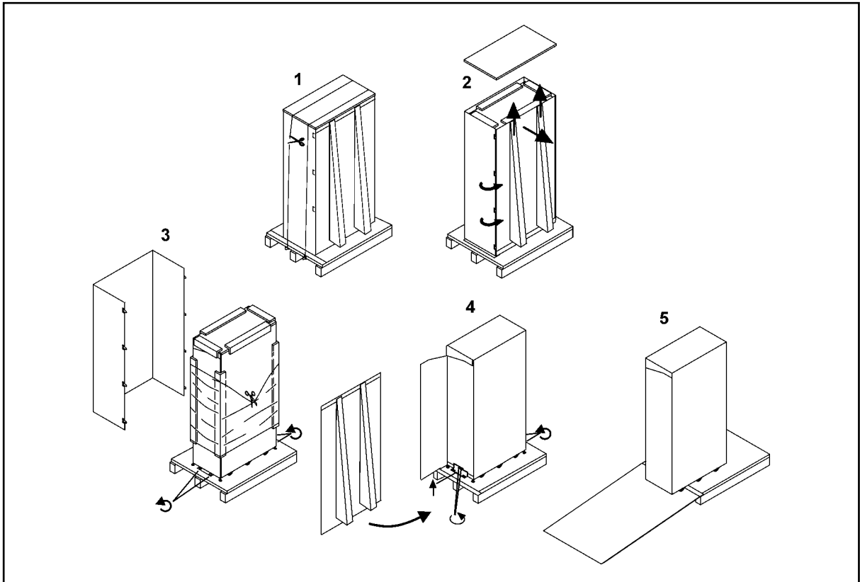
Abb. 3 Abnehmen der Anlage von der Palette
